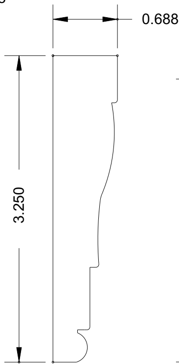
MB 606 (3-1/4 x 11/16)
