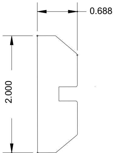
MB 4025 (2 x 11/16)
