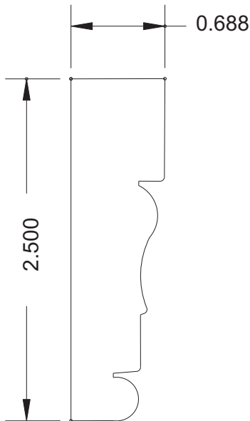
MB 6047 2-1/2 x 11/16
