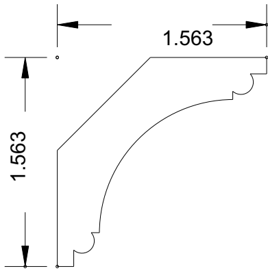
MB 1025 (2-1/4 x 11/16)
