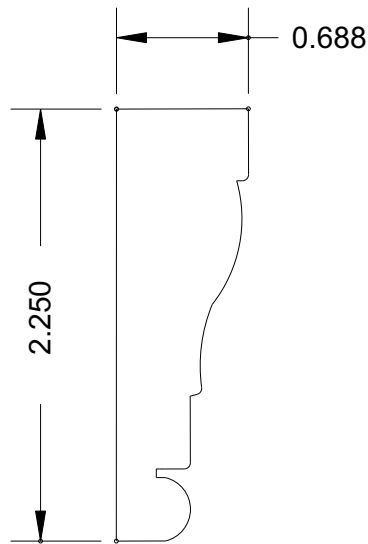
MB 6051 (2-1/4 x 11/16)
