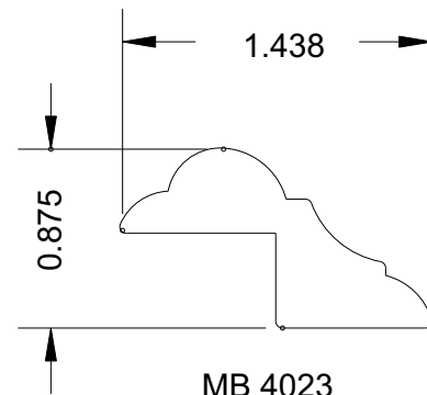
MB 4023 (1-1/2 x 5/8)
