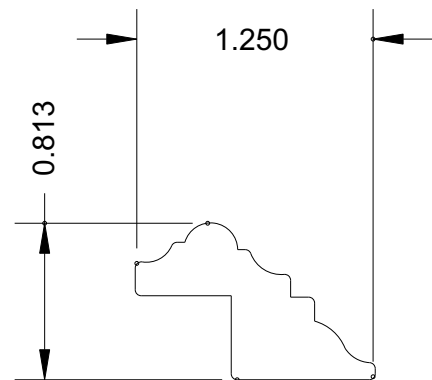
MB 4027 (1-1/4 x 9/16)
