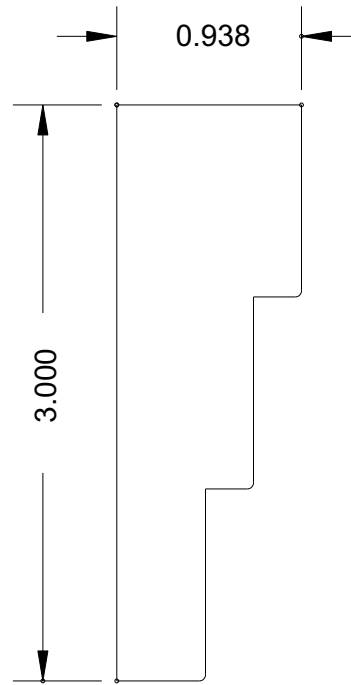
MB 607 (3 x 15/16)
