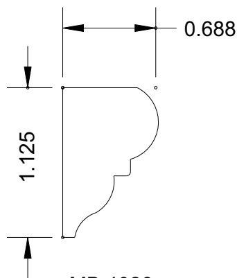
MB 4026 (1-1/8 x 11/16)
