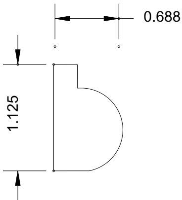
MB 855 (1-1/8 x 11/16)
