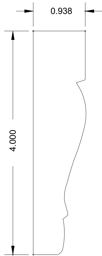
MB 6052 (4 x 15/16)
