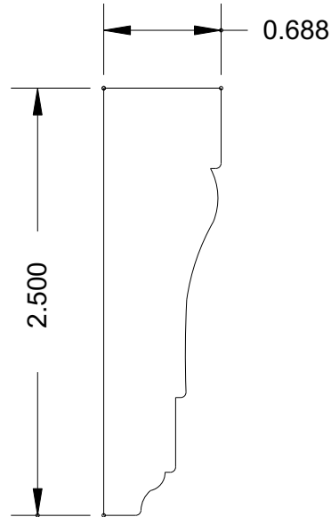
MB 658 (2-1/2 x 11/16)
