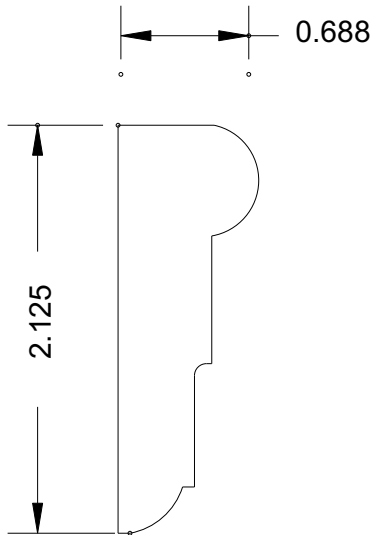
MB 844 (2-1/8 x 11/16)
