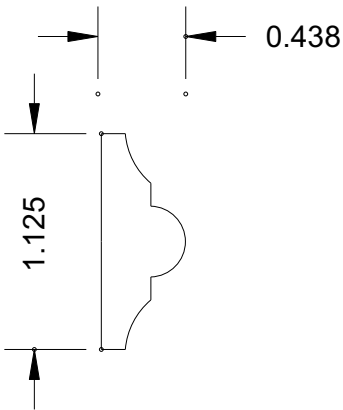
MB 787 (1-1/8 x 7/16)
