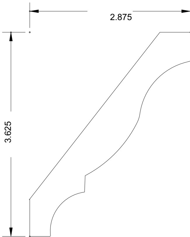
MB 125 (4-5/8 x 11/16)
