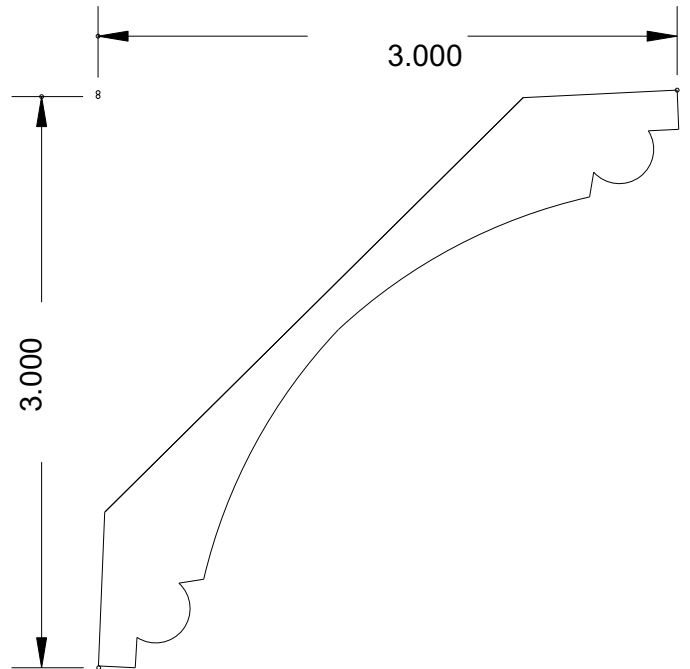
MB 156 (4-1/4 x 11/16)
