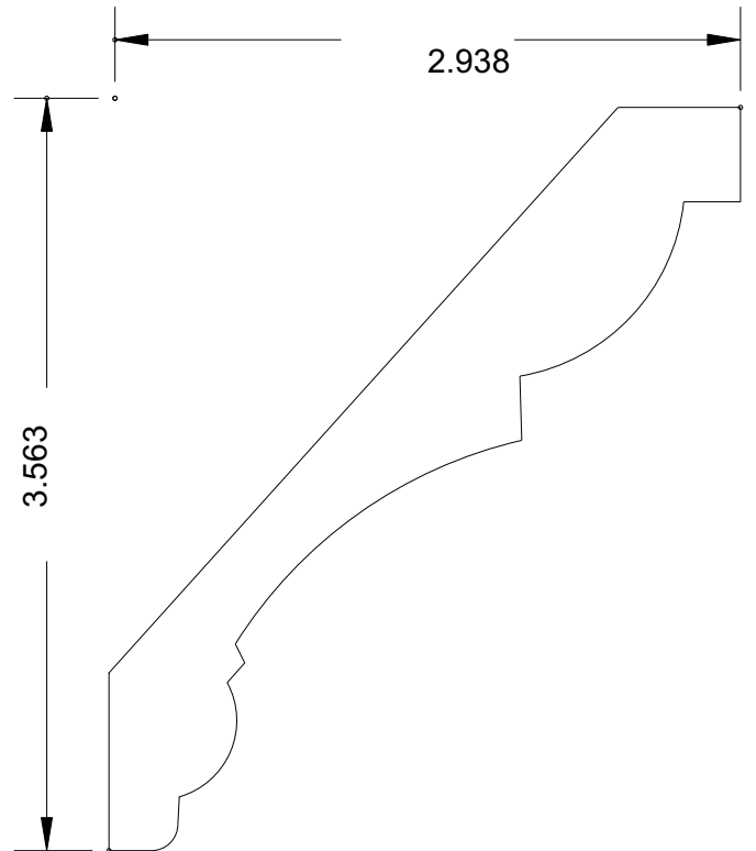
MB 168 (4-5/8 x 11/16)
