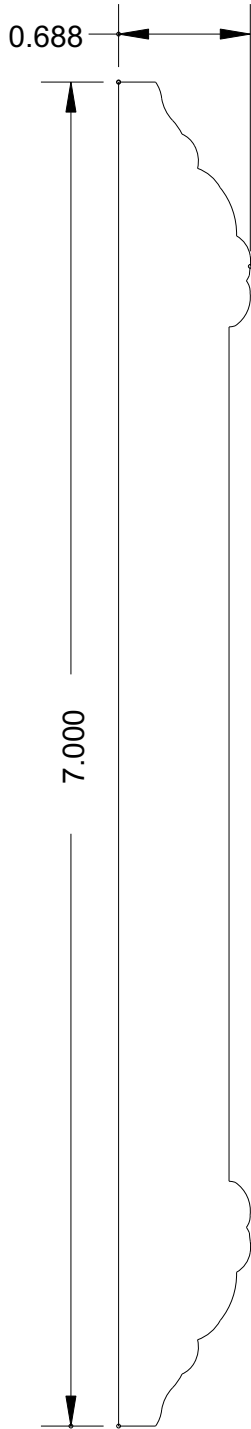
MB 959 (7 x 11/16)
