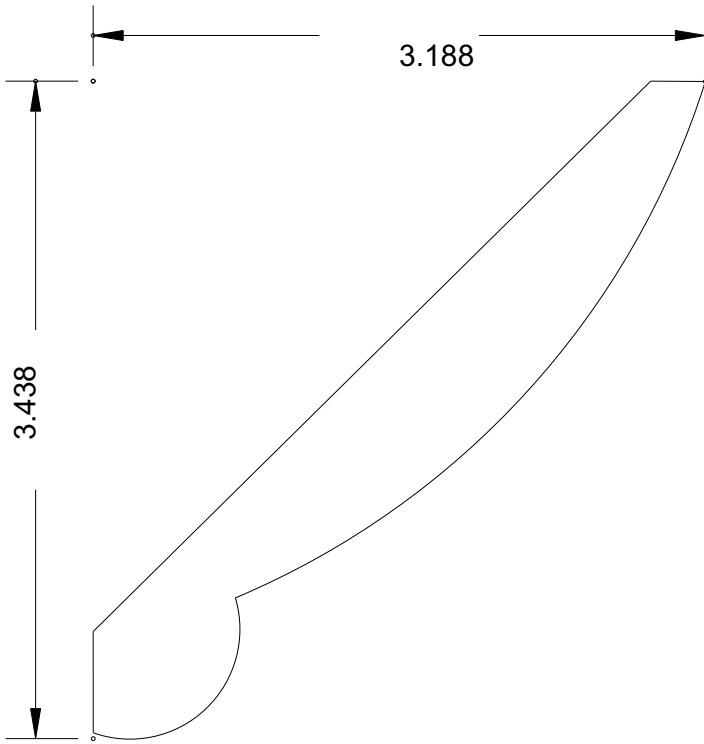
MB 120 (4-5/8 x 11/16)
